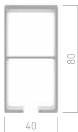
Perfil guía
