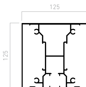
Viga guía 125x125 mm
